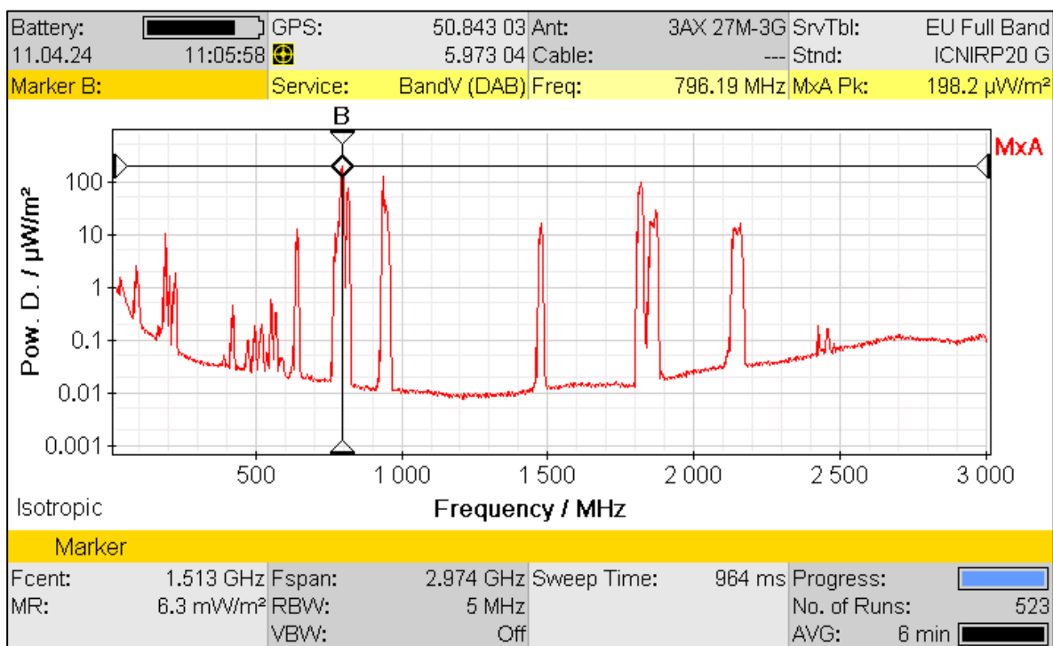
Figuur 3: Schermafbeelding van de selectieve EMV-meting
