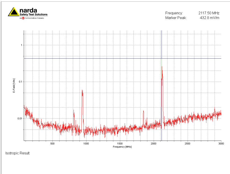
Figuur 1; Selectieve veldsterkte meting ingezoomd op sterkst aanwezige signaal, 2117.5 MHz (UMTS)
