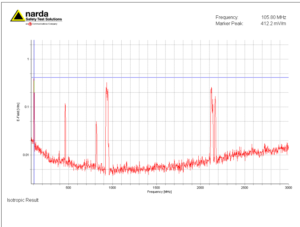
Figuur 1; Selectieve veldsterkte meting ingezoomd op sterkst aanwezige signaal, 105.8 MHz (FM-omroep)
