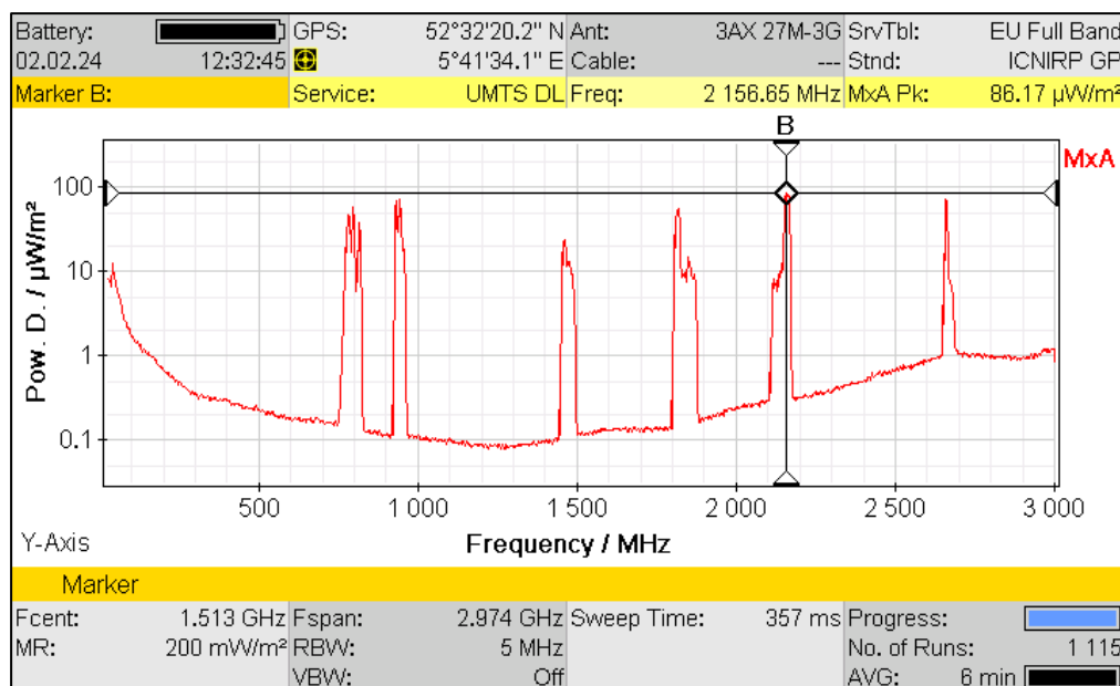
Figuur 4: Plot van de selectieve EMV-meting
