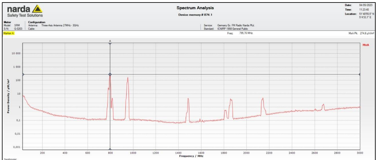
Figuur 12: Plot van de selectieve EMV-meting, keuken
