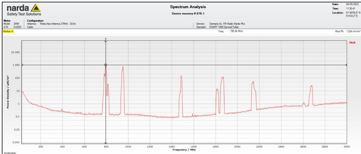
Figuur 13: Plot van de selectieve EMV-meting, tuin
