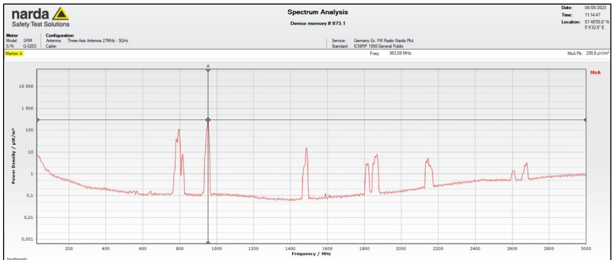
Figuur 11: Plot van de selectieve EMV-meting, kinderkamer
