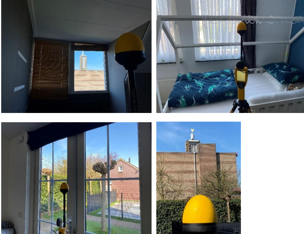
Figuur 1 tot en met 4: Foto's van de breedbandige outdoor en indoor meetopstelling
