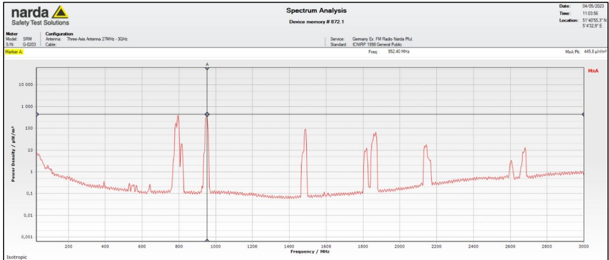
Figuur 10: Plot van de selectieve EMV-meting, zolder.
