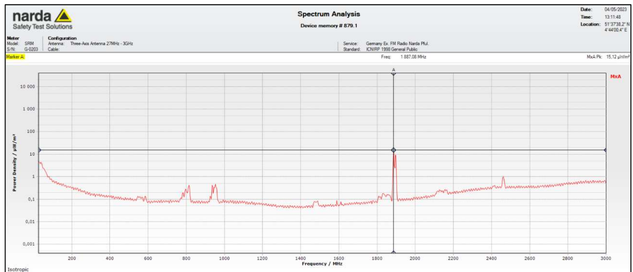
Figuur 6: Plot van de selectieve EMV-meting, woonkamer
