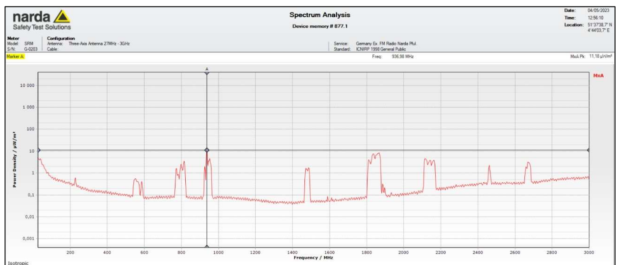
Figuur 7: Plot van de selectieve EMV-meting, tuin
