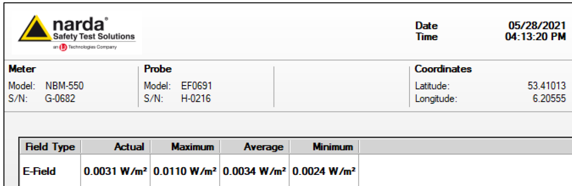
Figuur 4: Plot van de breedbandige EMV-meting
