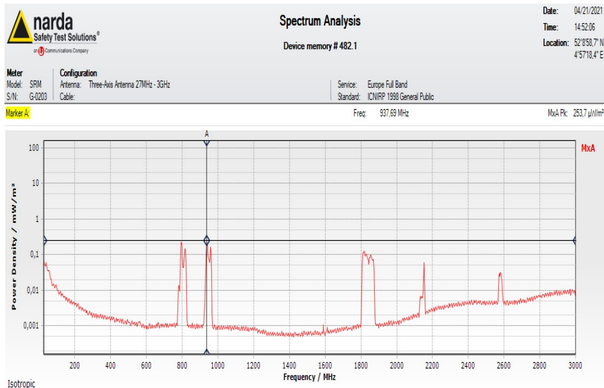
Figuur 4: Plot van de selectieve EMV-meting
