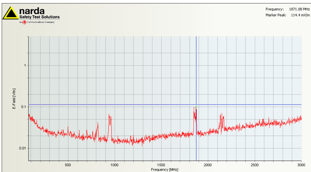
Figuur 1; Selectieve veldsterkte meting hoek IJweg thv.Kleine Belt, ingezoomd op sterkst aanwezige signaal, 1871.88 MHz (DCS1800)
