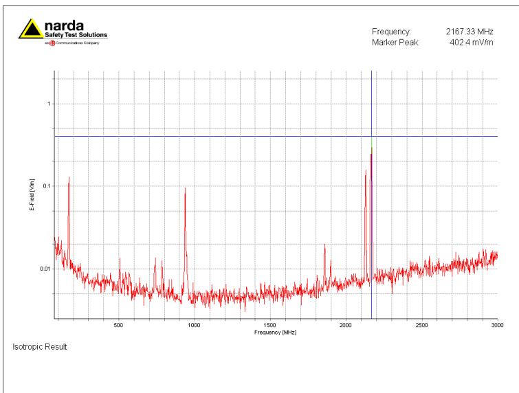
Figuur 1; Selectieve veldsterkte meting ingezoomd op sterkst aanwezige signaal, 2167.3 MHz (UMTS)
