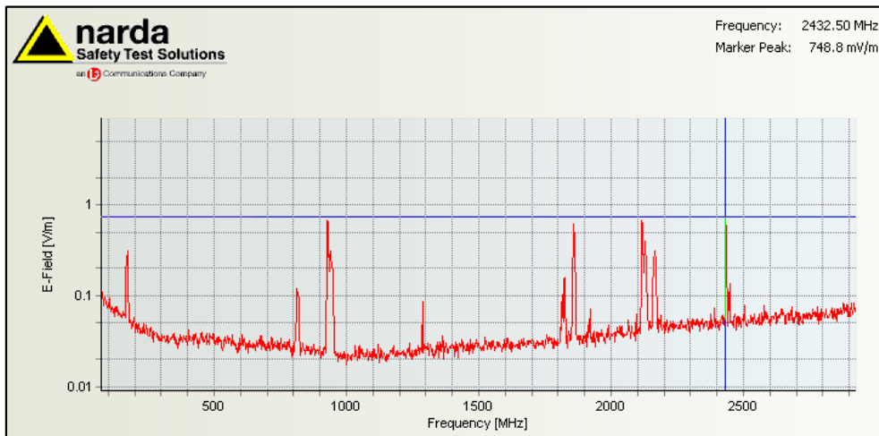
Figuur 1; Selectieve veldsterkte meting ingezoomd op sterkst aanwezige signaal, 2432.50 MHz, WLAN.
