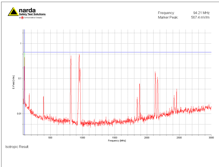
Figuur 1; Selectieve veldsterkte meting ingezoomd op het sterkst aanwezige signaal, 94.2 MHz (FM-omroep)
