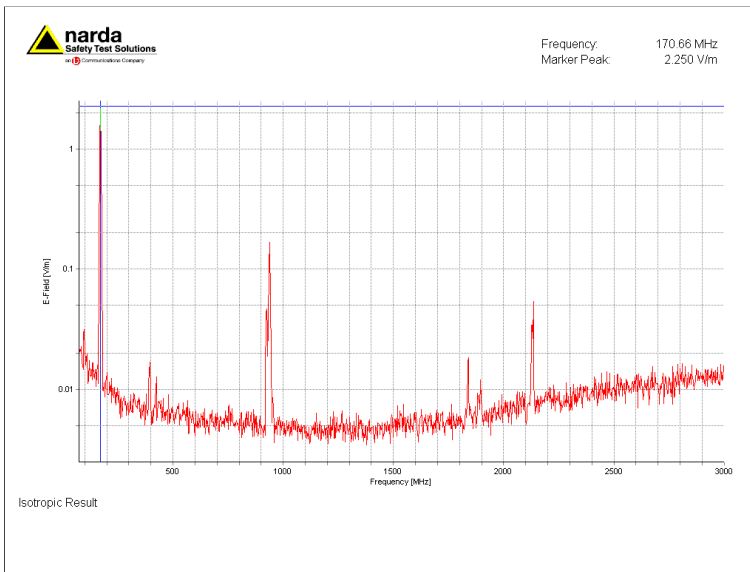
Figuur 1; Selectieve veldsterkte meting ingezoomd op sterkst aanwezige signaal, 170.66 MHz (P-2000)
