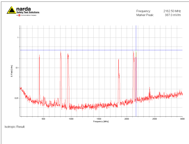
Figuur 1; Selectieve veldsterkte meting ingezoomd op sterkst aanwezige signaal, 2162.5 MHz (UMTS)
