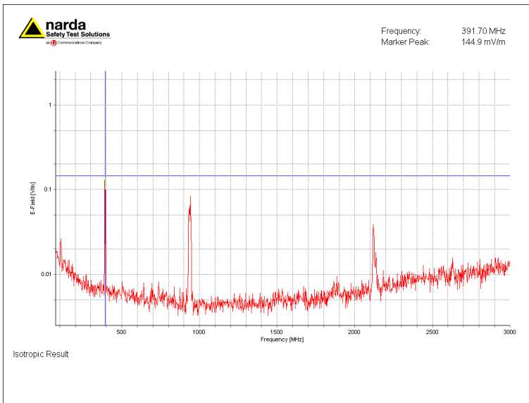
Figuur 1; Selectieve veldsterkte meting ingezoomd op sterkst aanwezige signaal, 391.7 MHz (C-2000)
