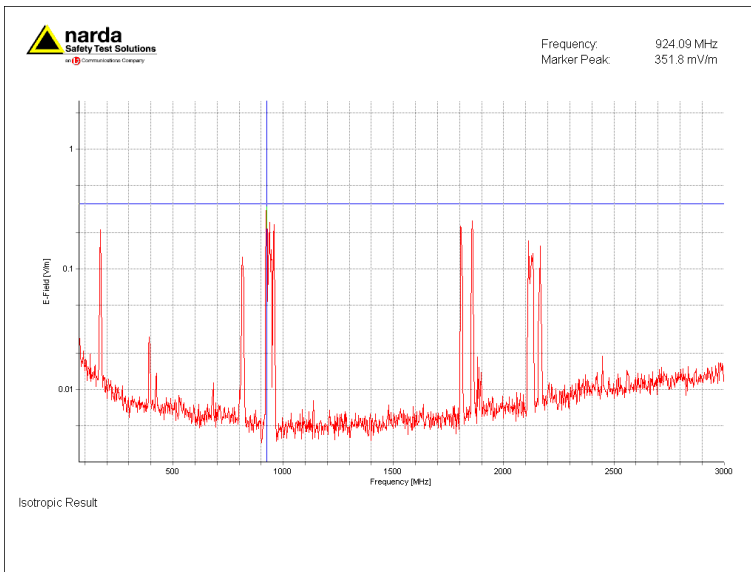
Figuur 1; Selectieve veldsterkte meting ingezoomd op het sterkst aanwezige signaal, 924 MHz (GSM-900)
