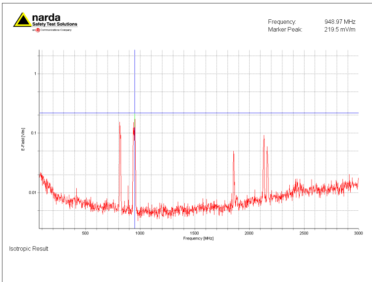
Figuur 1; Selectieve veldsterkte meting ingezoomd op het sterkst aanwezige signaal, 948.9 MHz (GSM-900)
