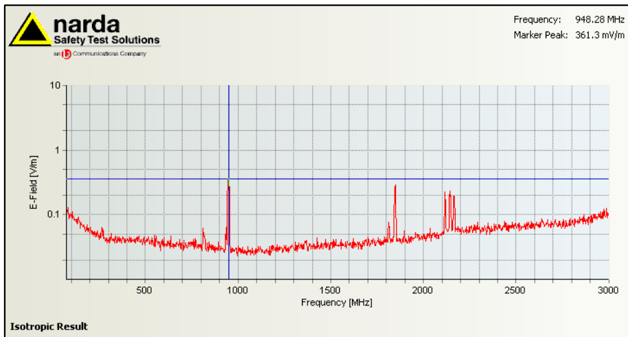
Figuur 1; Selectieve veldsterkte meting ingezoomd op sterkst aanwezige signaal, 948.28 MHz, GSM.
