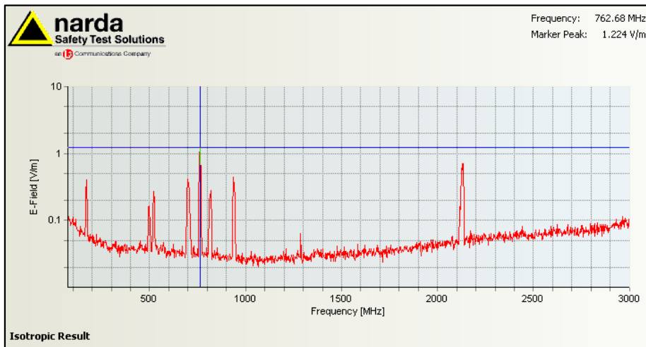
Figuur 1; Selectieve veldsterkte meting ingezoomd op sterkst aanwezige signaal, 762.68 MHz, DVB-T.
