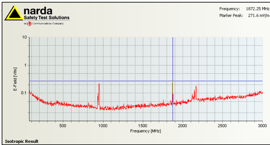
Figuur 1; Selectieve veldsterkte meting ingezoomd op sterkst aanwezige signaal, 1872.25 MHz, DCS (GSM1800).
