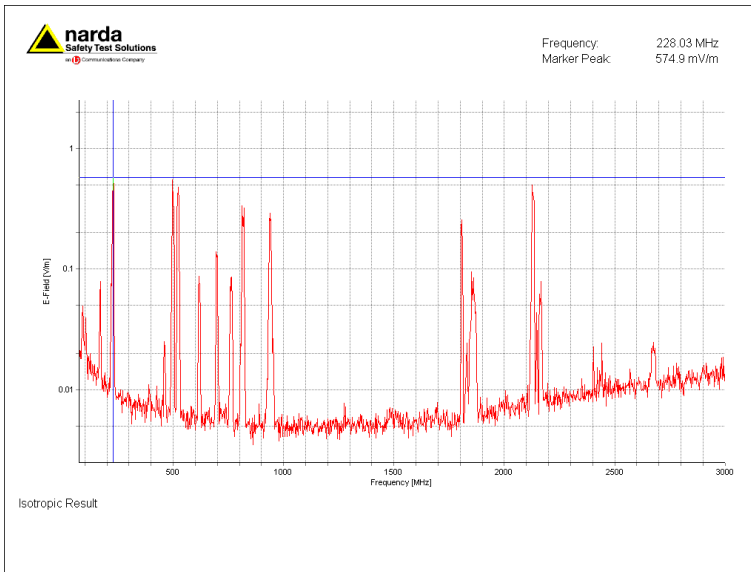
Figuur 1; Selectieve veldsterkte meting ingezoomd op sterkst aanwezige signaal, 228.03 MHz (DAB)
