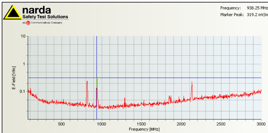
Figuur 1; Selectieve veldsterkte meting ingezoomd op sterkst aanwezige signaal, 938.25 MHz, GSM.
