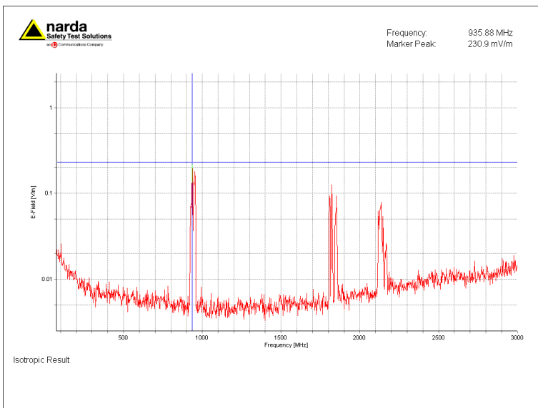
Figuur 1; Selectieve veldsterkte meting ingezoomd op sterkst aanwezige signaal, 935.8 MHz (GSM-900)
