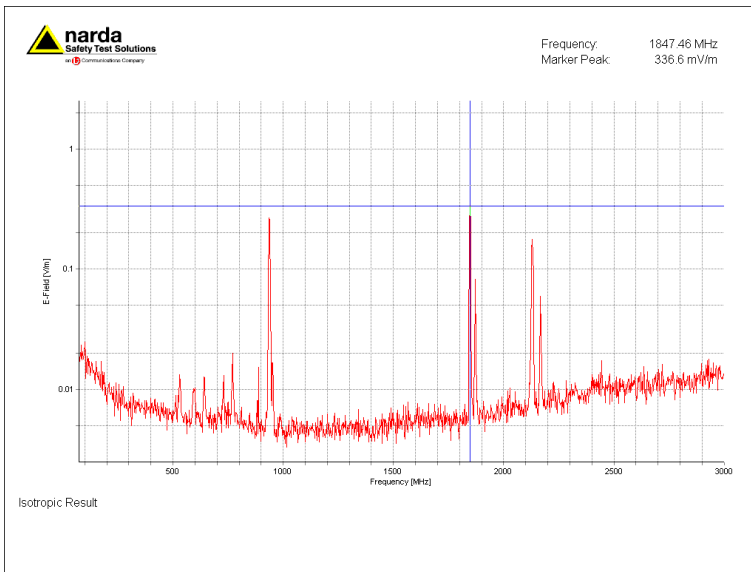
Figuur 1; Selectieve veldsterkte meting ingezoomd op het sterkst aanwezige signaal, 1847.4 MHz DCS(GSM1800)
