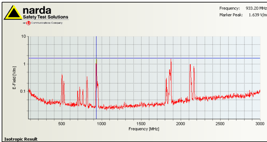
Figuur 1; Selectieve veldsterkte meting ingezoomd op sterkst aanwezige signaal, 933.20 MHz, GSM.
