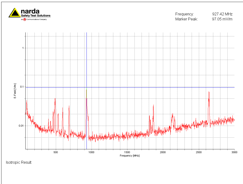
Figuur 1; Selectieve veldsterkte meting ingezoomd op sterkst aanwezige signaal, 927.4 MHz (GSM)
