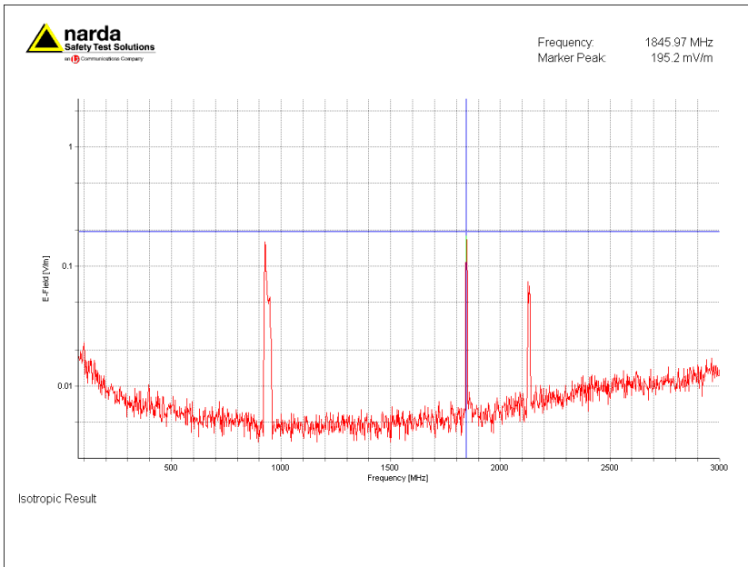
Figuur 1; Selectieve veldsterkte meting ingezoomd op sterkst aanwezige signaal, 1845.9 MHz (DCS(GSM1800))
