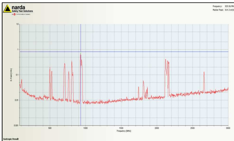
Figuur 1; Selectieve veldsterkte meting ingezoomd op sterkst aanwezige signaal, 929.56 MHz, GSM.
