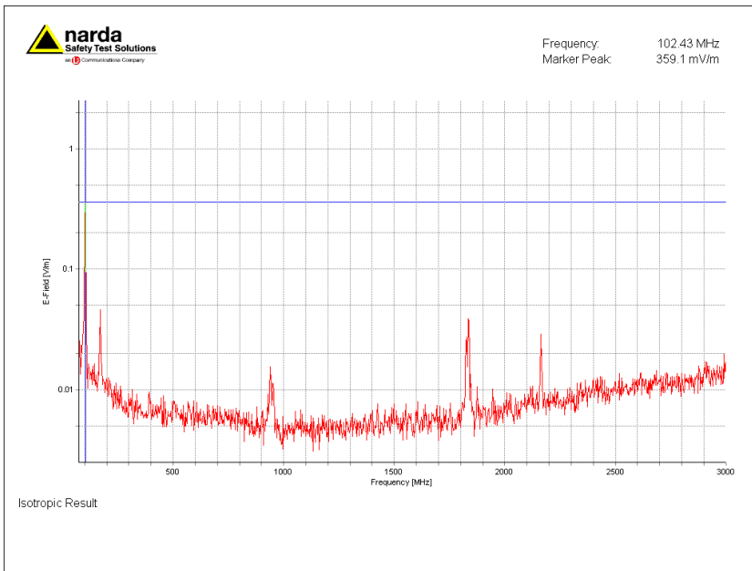
Figuur 1. Selectieve veldsterkte meting ingezoomd op sterkst aanwezige signaal, 102.4 MHz (FM-omroep)
