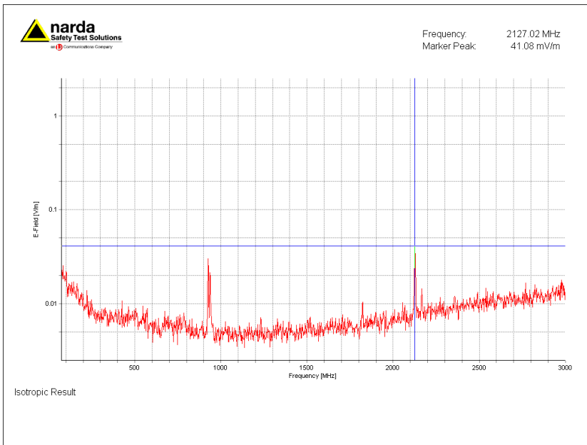
Figuur 1; Selectieve veldsterkte meting ingezoomd op sterkst aanwezige signaal, 2127.0 MHz (UMTS)
