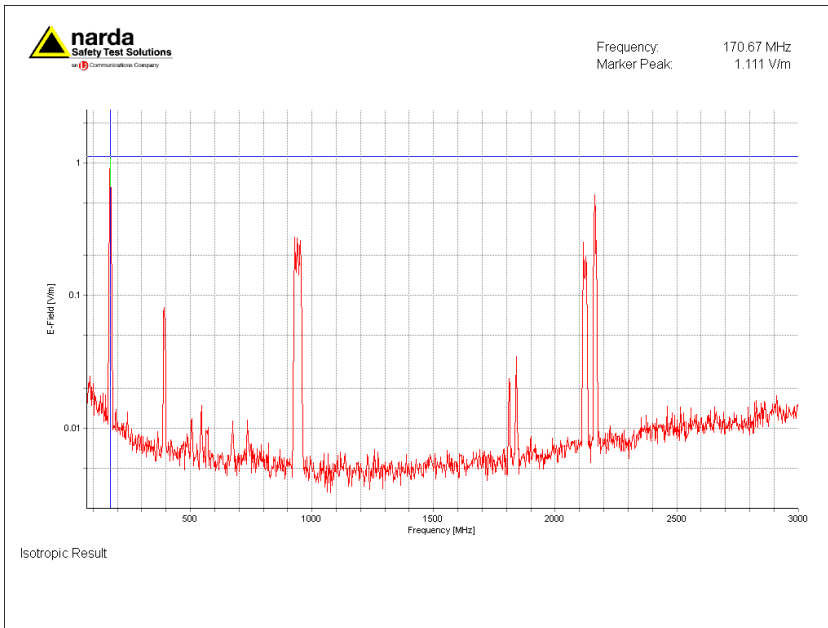
Figuur 1. Selectieve veldsterkte meting ingezoomd op sterkst aanwezige signaal, 170.6 MHz (P-2000)
