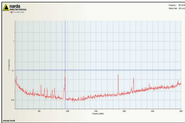
Figuur 1; Selectieve veldsterkte meting ingezoomd op sterkst aanwezige signaal, 926.49 MHz, GSM.
