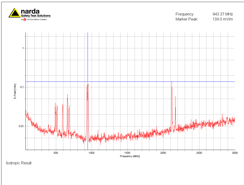
Figuur 1; Selectieve veldsterkte meting ingezoomd op sterkst aanwezige signaal, 943.3 MHz (GSM900)
