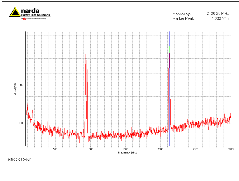
Figuur 1. Selectieve veldsterkte meting ingezoomd op sterkst aanwezige signaal, 2130.2 MHz (UMTS)
