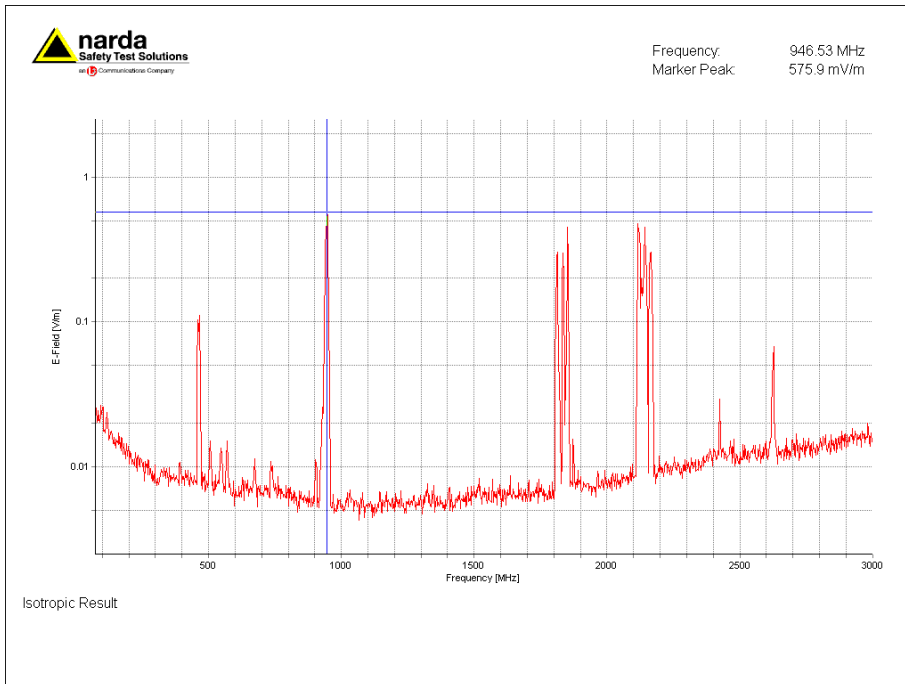
Figuur 1. Selectieve veldsterkte meting ingezoomd op sterkst aanwezige signaal, 946.5 MHz (GSM)
