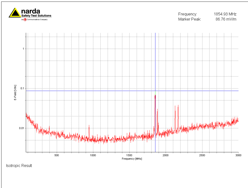
Figuur 1; Selectieve veldsterkte meting ingezoomd op sterkst aanwezige signaal, 1854.9 MHz (DCS(GSM)1800)
