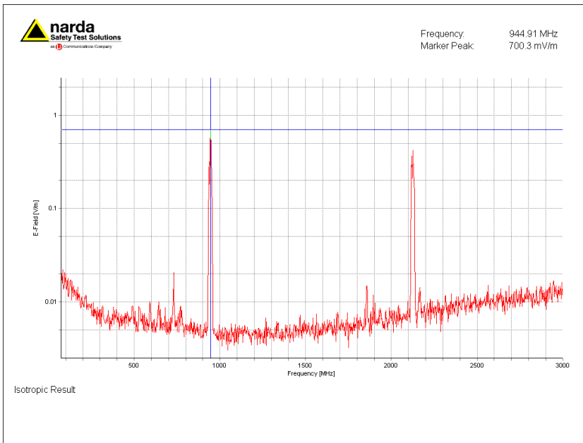
Figuur 1; Selectieve veldsterkte meting ingezoomd op sterkst aanwezige signaal, 944.9 MHz (GSM)
