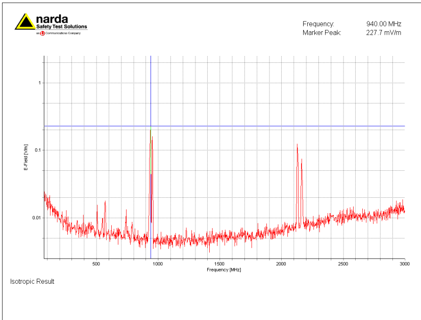
Figuur 1. Selectieve veldsterkte meting ingezoomd op sterkst aanwezige signaal, 940.0 MHz (GSM)
