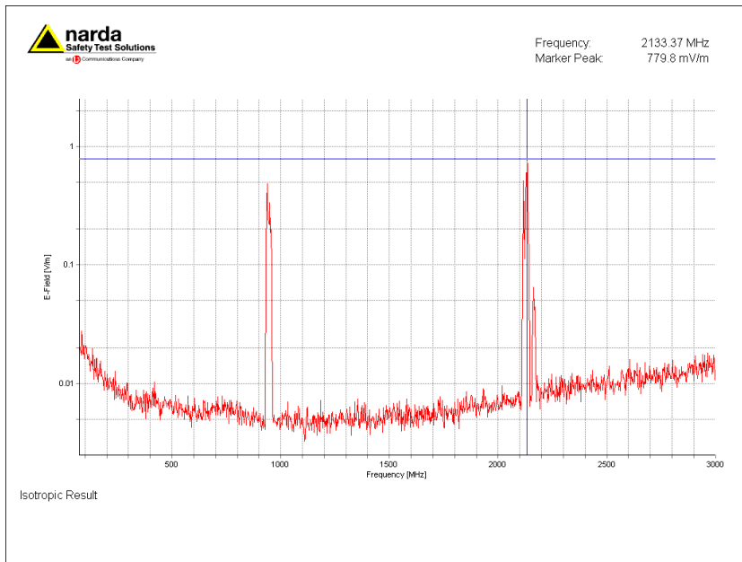
Figuur 1; Selectieve veldsterkte meting ingezoomd op sterkst aanwezige signaal, 2133.3 MHz (UMTS)
