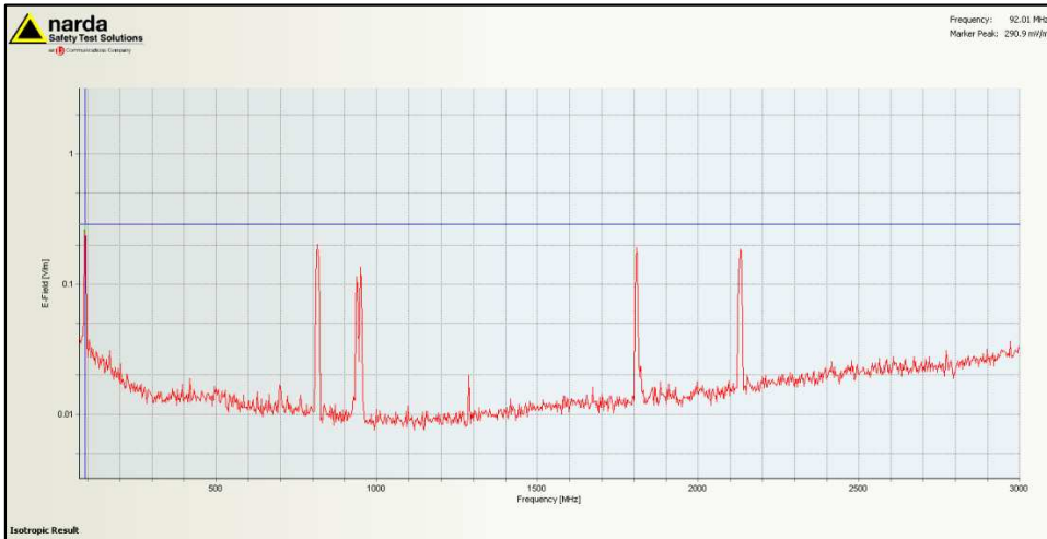
Figuur 1; Selectieve veldsterkte meting ingezoomd op sterkst aanwezige signaal, 92.01 MHz, FM omroep
