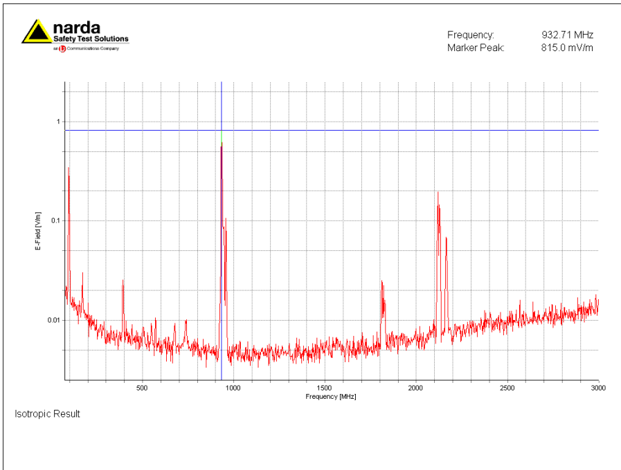
Figuur 1. Selectieve veldsterkte meting ingezoomd op sterkst aanwezige signaal, 932.7 MHz (GSM)
