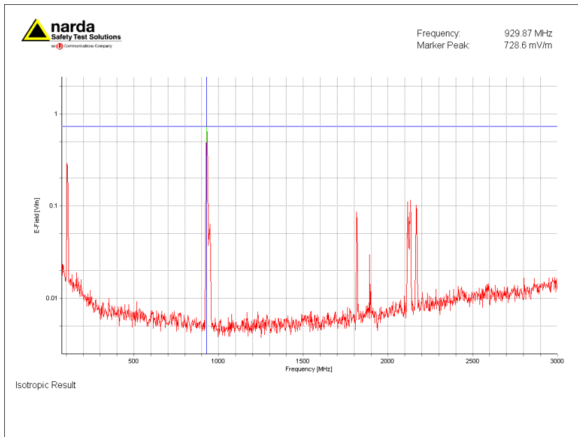
Figuur 1; Selectieve veldsterkte meting ingezoomd op sterkst aanwezige signaal, 929.8 MHz (GSM900)
