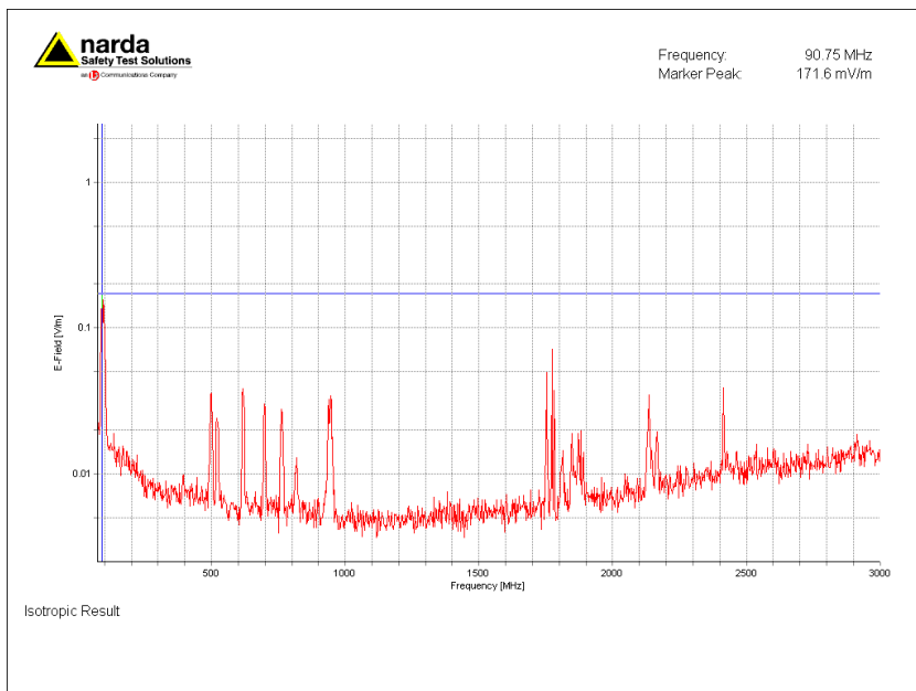
Figuur 1; Selectieve veldsterkte meting ingezoomd op sterkst aanwezige signaal, 90,7 MHz (FM-omroep)
