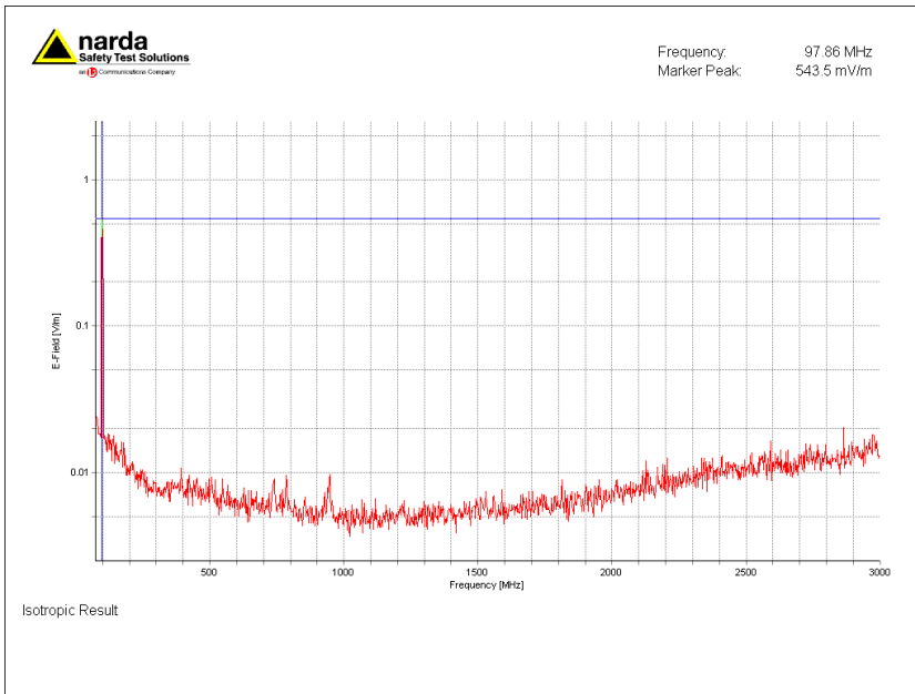
Figuur 1. Selectieve veldsterkte meting ingezoomd op sterkst aanwezige signaal, 97.8 MHz (FM-omroep)
